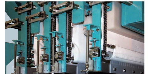
3 移動ろ布はエンドレス構造のチェーンに取り付けられ、回転とスクレーパーによりケーキを剥離します。
